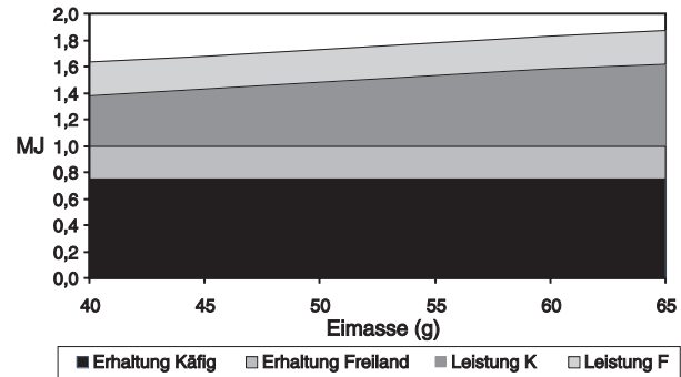
Abbildung 1: Energiebedarf von Legehennen (1800 g Körpergewicht in Käfighaltung, 2200 g Körpergewicht in Freilandhaltung)
